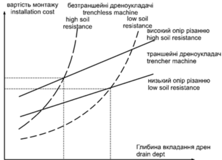
Рис. 3. Порівняння питомої вартості вкдання дренажу від глибини дрен траншейним способом та дренажкдачем V-подібної конструкції [12]
