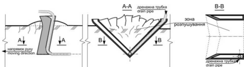
Рис. 2. Ніж V-подібної конструкції (V-Plow): а) на дрепоукладачі фірми Mastenbroek; б) схема різання ґрунту, види ззаду та збоку
