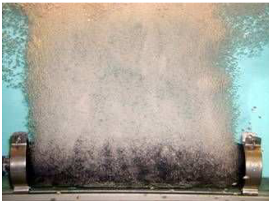
Рис. 3. Донний аератор
