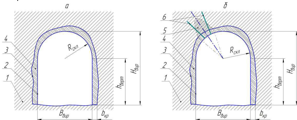
Рис. 3. Переріз підземної транспортної виробки пройденної в: а – стійкому масиві; б – нестійкому масиві; 1 – гірський масив; 2 – контур виробки у світлі; 3 – контур виробки в проходці; 4 – бетонне (залізобетонне) кріплення; 5 – зона вивалоутворення; 6 – анкер
