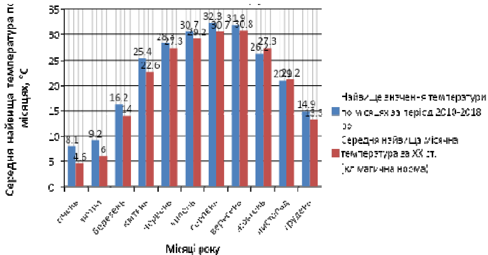
Рис. 3. Порівняльна діаграма динаміки максимальної температури повітря досліджуваного періоду на ст. Любешів та кліматичної норми ХХ ст.
