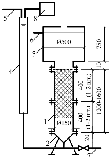
Рис. 2.2. Експериментальна установка для дослідження безнапірного знезалізнення води
