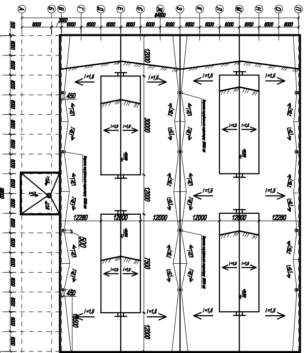
План покрівлі (1:400)
