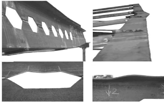
Рис. 1. Втрата місцевої стійкості елементів перерізу прогону
