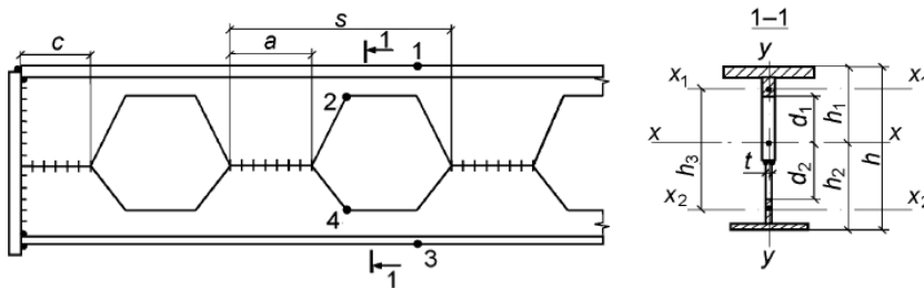
Рис. 2. Схема ділянки балки з перфорованою стінкою
