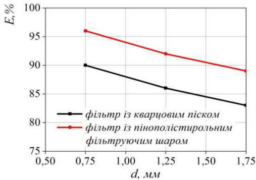
Рис. 4. Ефективність очищення води від органічних речовин при різних діаметрах гранул ( H = 1,0 м, V = 2 м/год, перманганатна окислюваність = 35 \text{ мгO}_2/\text{дм}^3 , фільтроцикл № 5...10)
