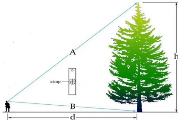
Рисунок 6.1. Визначення висоти дерева за допомогою базисного висотоміра
