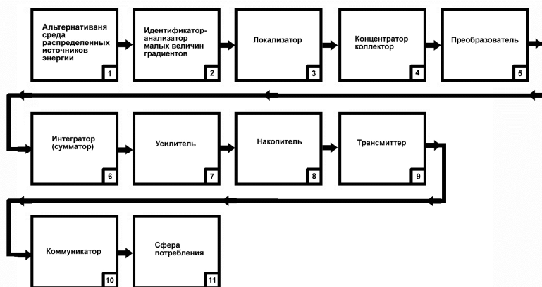
Рис. 1. Макроструктурная алгоритмическая модель градиентного электрогенератора
