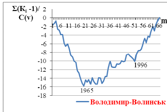
Рис. 2. Різницеві інтегральні криві сум атмосферних опадів за рік деяких метеостанцій Західного Полісся та Волині
