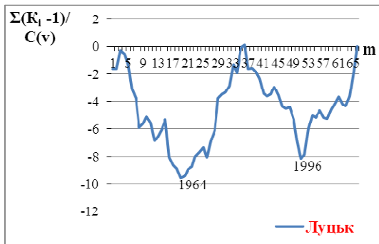
Рис. 2. Різницеві інтегральні криві сум атмосферних опадів за рік деяких метеостанцій Західного Полісся та Волині
