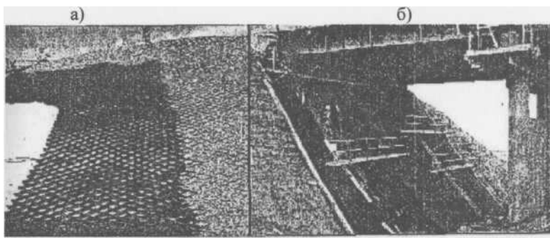
Рис. 2. Різні варіанти армуючих систем підводного і надводної частин укосів: а) георешітка заповнюється фракціями щебеню; б) георешітка, чарунки якої заповнені бетоном
