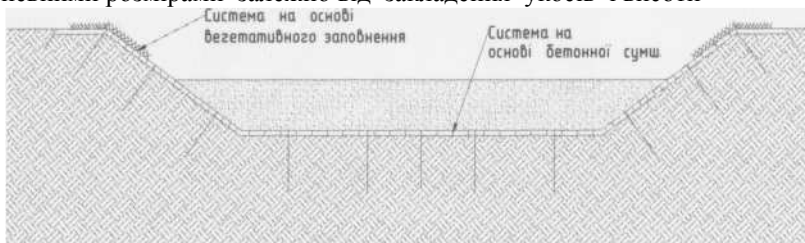
Рис. 6. Конструктивне рішення цементобетонного захисту
