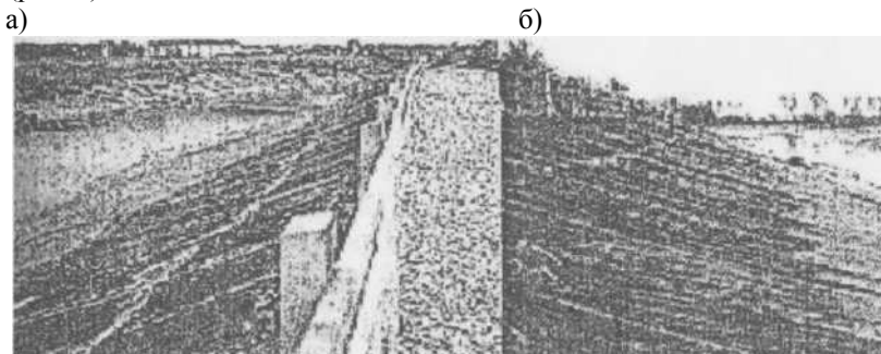
Рис. 1. Берегоукріплювальні заходи: а) габійні конструкції; б) сітчасті конструкції
