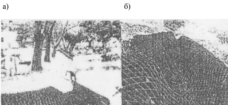
Рис. 3. Різні варіанти використання георешіток: а) захист берега від розмиву; б) зміцнення русла малих водотоків
