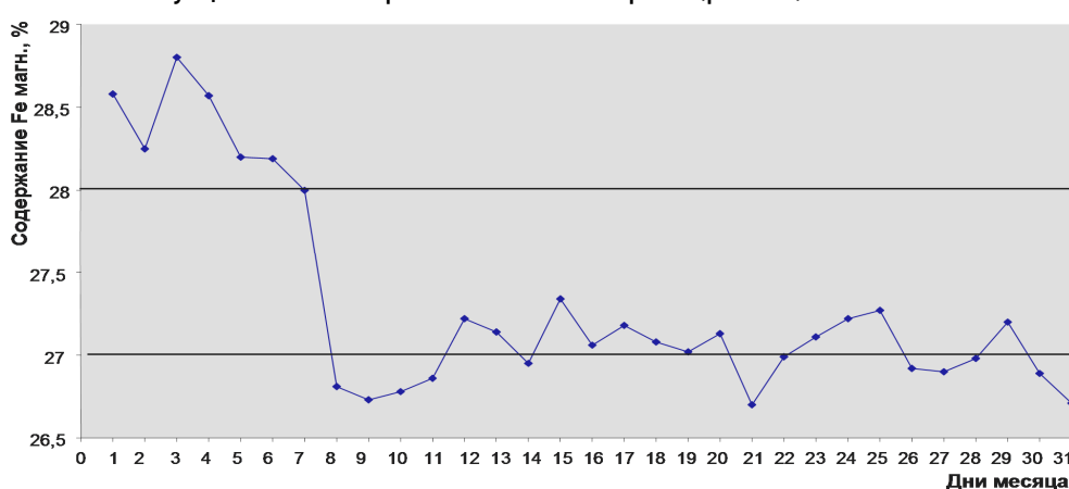
Рис. 2. Колебания содержания железа магнитного в рудопотоке карьера №3 ГД ПАО «АрселорМиттал Кривой Рог» за январь месяц 2012 г.
