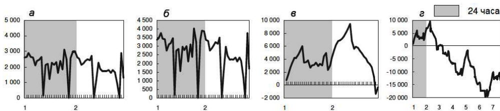
Рис. 3. Характер пульсаций реальной загрузки тракта ЦПТ ИнГОКа
