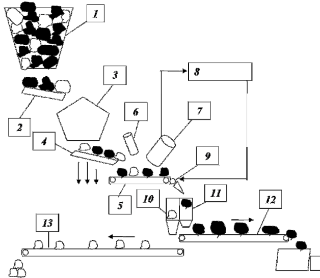
Рис. 5. Функциональная схема мобильного дробильно-сортировочного радиометрического комплекса
