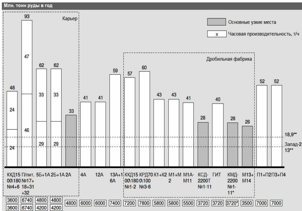
Рис. 4. Технический лимит оборудования западного тракта ИнГОКа
