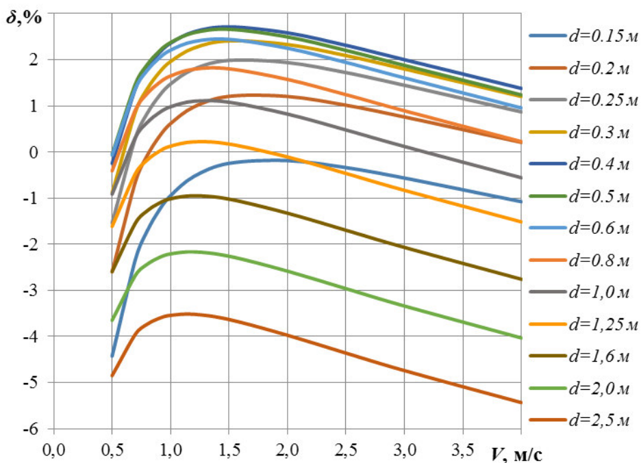
Рис. 2. Похибки розрахунків гідравлічних уклонів за формулою (7) у порівнянні із розрахунками за формулами (4) і (5) (Федорова М.Ф.)
